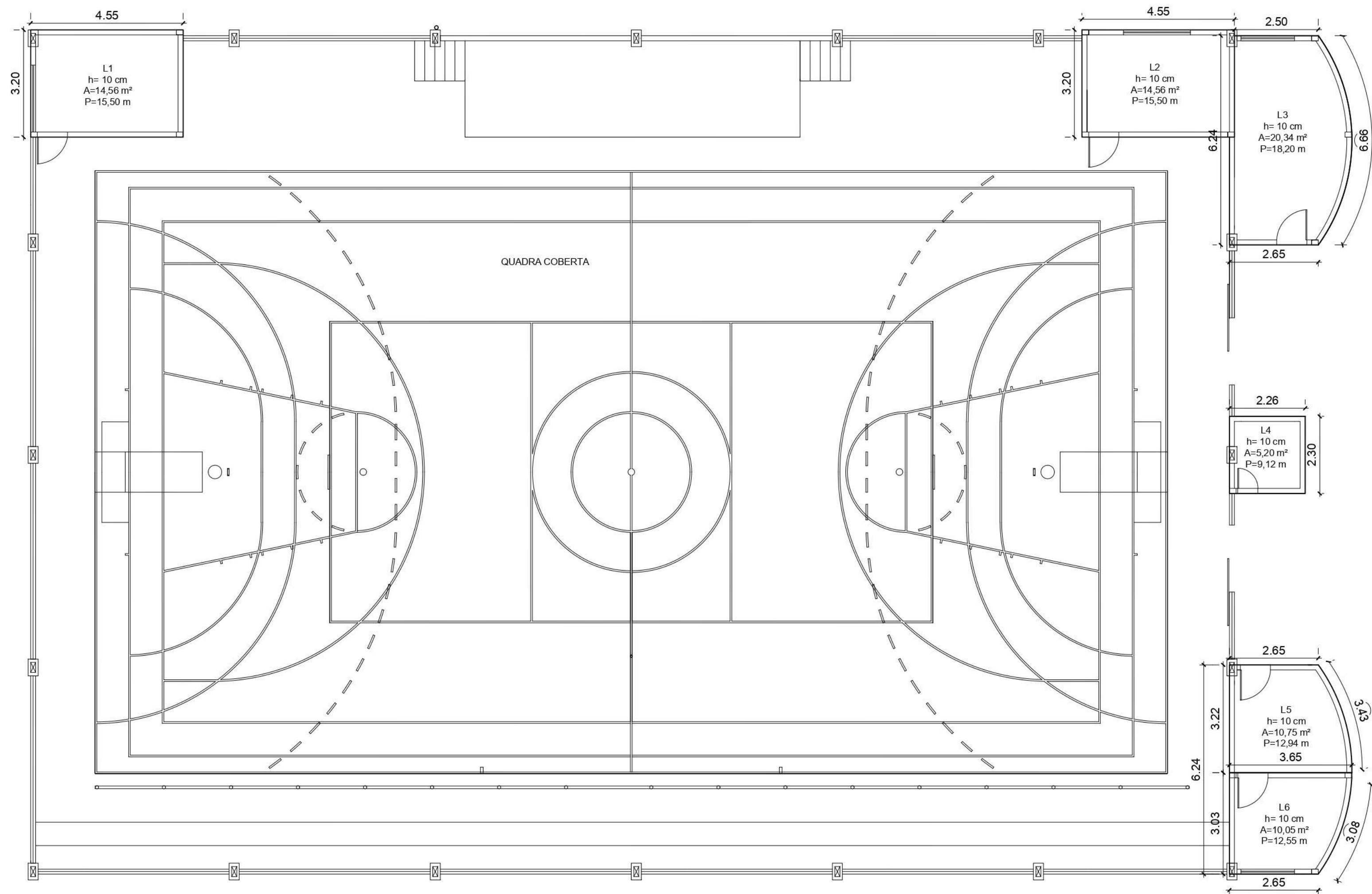
INDICAÇÃO DE LAJES ESCALA 1/100
