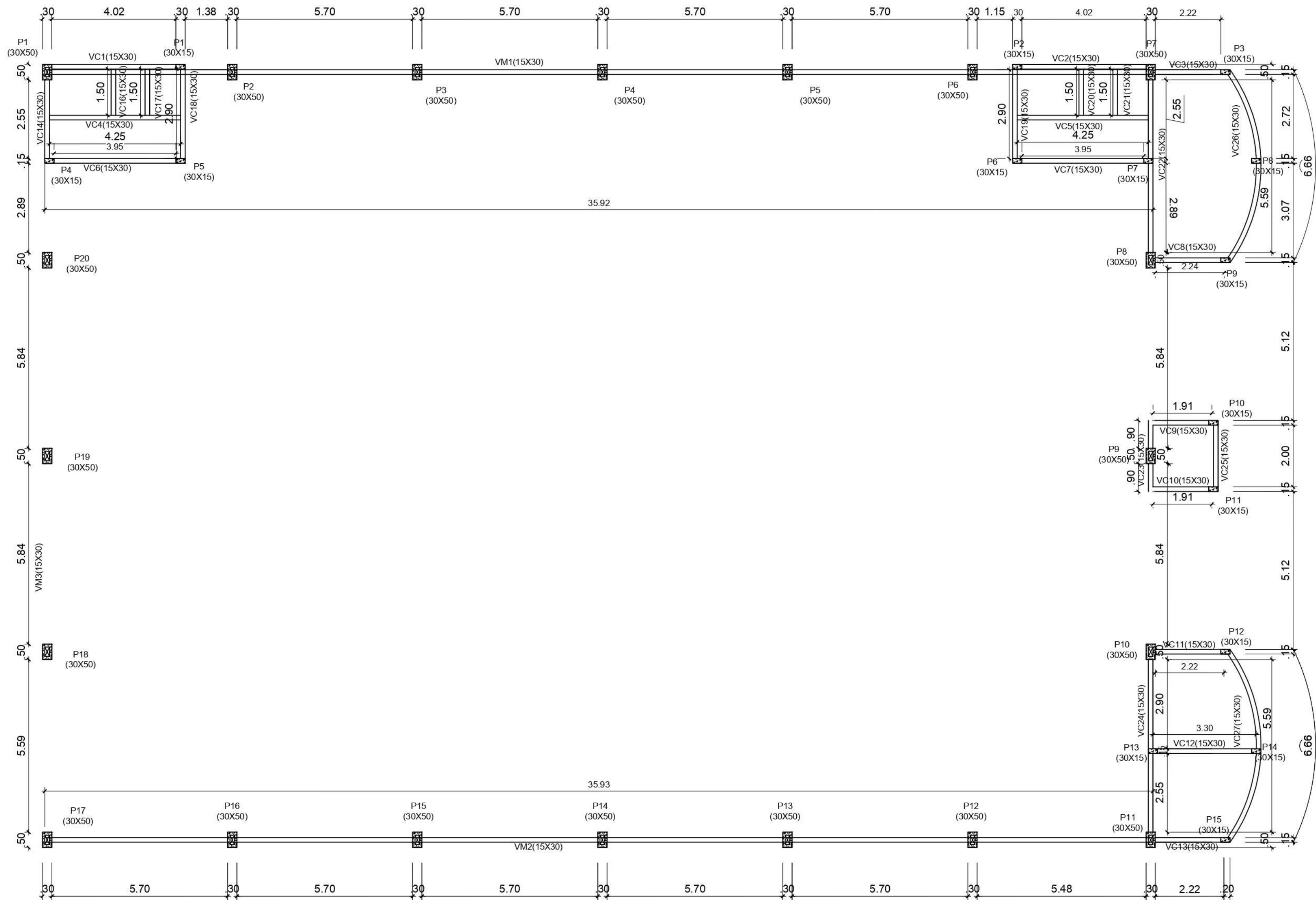
SUPRAESTRUTURA ESCALA 1/100
