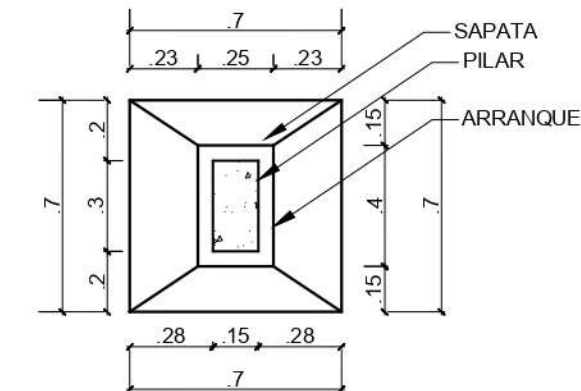
SAPATA 15 UNIDADES (S2) SAPATAS ESCALA 1/25
