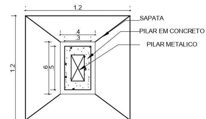
SAPATA 20 UNIDADES (S1) SAPATAS ESCALA 1/25
