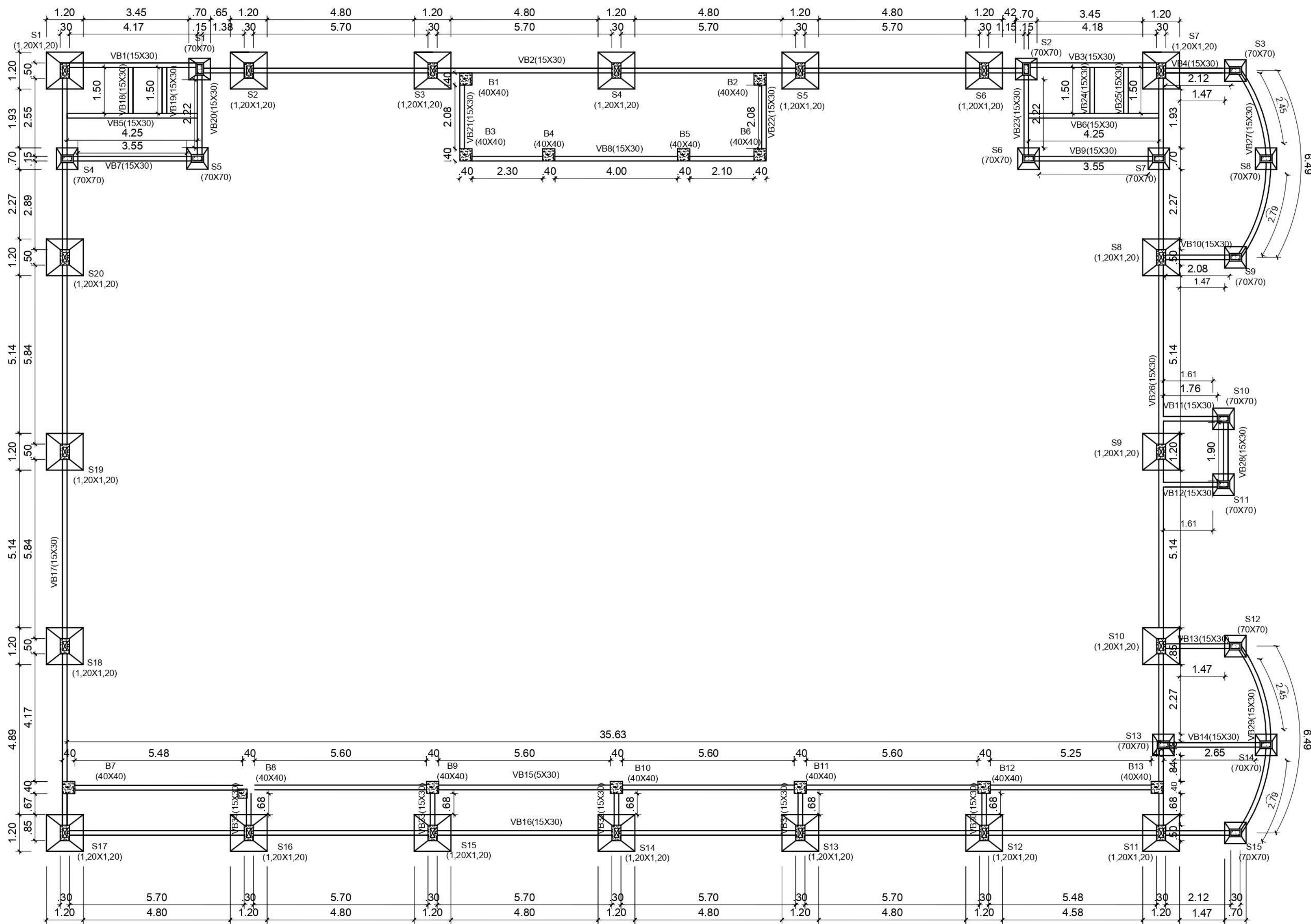
INFRAESTRUTURA ESCALA 1/100
