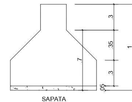
SAPATA 15 UNIDADES (S2) SAPATAS ESCALA 1/25
